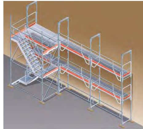
Échafaudage de pied
